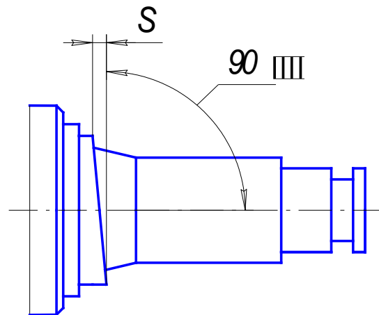
Схема измерения величины бокового биения заплечика вала.
